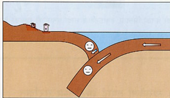
चित्र नं. ३- समुन्द्रमा चुनामी कसरी उब्जिन्छ भन्ने जानकारी
