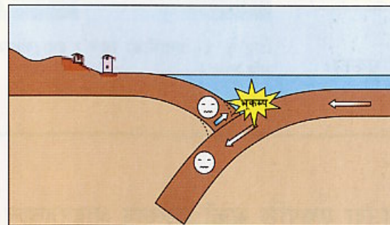
चित्र नं. २- टेक्टोनिक प्लेटहरूबीचका सीमानाहरू तथा भूगर्भ भित्रको अन्तर्कृया
